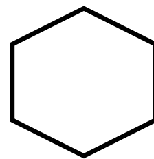
环己烷 ( C_6H_{12} )
